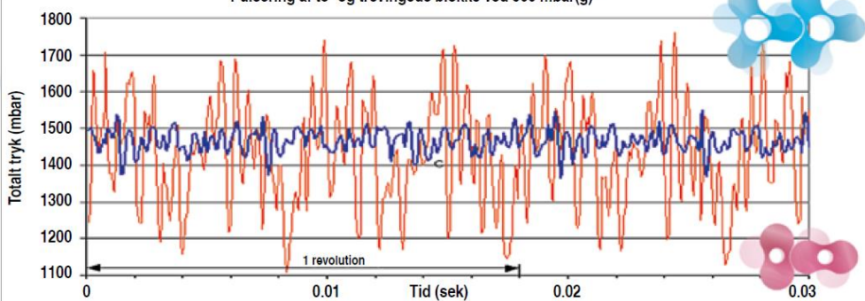
Pulsering af to- og trevingede blokke ved 500 mbar(g)
